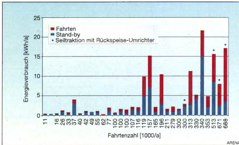
Bild 4 Stand-by- und Fahrten-Energieverbrauch der Aufzüge nach Fahrtenzahl Fahrten-Verbrauch mit Formel 1 berechnet. Tiefer Fahrten-Verbrauch bei hoher Fahrtenzahl kann durch kleine Nennlast, Motorleistung und Hubhöhe bedingt sein. Es lassen sich keine einfachen Folgerungen ziehen.
