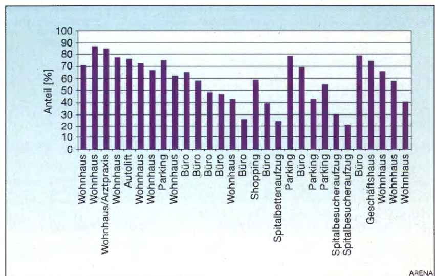
Bild 5 Anteil Stand-by am gesamten Energieverbrauch, nach Gebäudeart Gleiche Reihenfolge wie Bild 4. Anlagen mit einem Stand-by-Verbrauch von weniger als 30% sind Anlagen mit sehr hohen Fahrtenzahlen.
