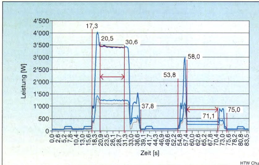
Bild 2 Messwerte der Leerfahrten eines Seilzugs mit Gegengewicht Dunkelblau: die Gesamtleistungsaufnahme; hellblau/hellgrün: die 3 Phasen; rot: die Hilfslinien zur Beurteilung der Fahrabschnitte.
