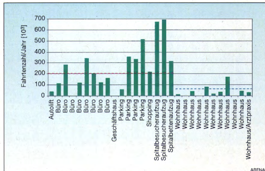
Bild 3 Fahrtenzahl der gemessenen Aufzüge nach Gebäudenutzung
