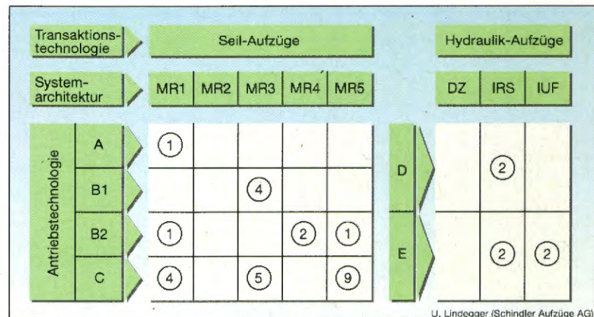
Bild 1 Gemessene Aufzüge in der Technologiematrix. Die Zahlen in den Kreisen geben die Anzahl der ausgemessenen Aufzüge an.
