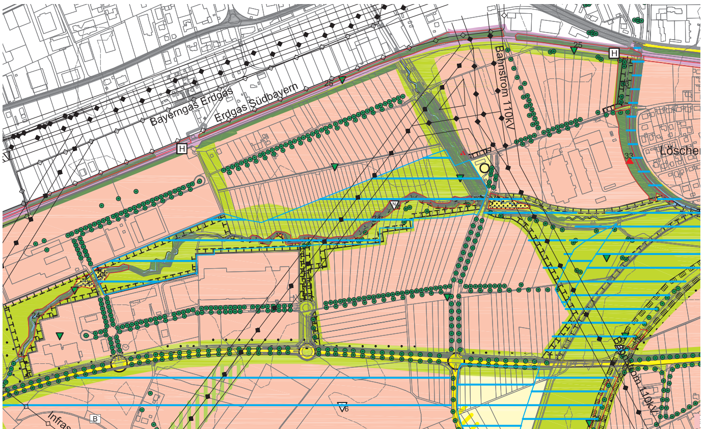
Änderung Landschaftsplan mit Deckblatt Nr. 27 im Bereich "Gewerbegebiet Münchnerau - An der Fuggerstraße"
