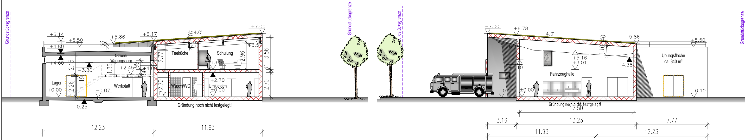
Schnitt D-D
