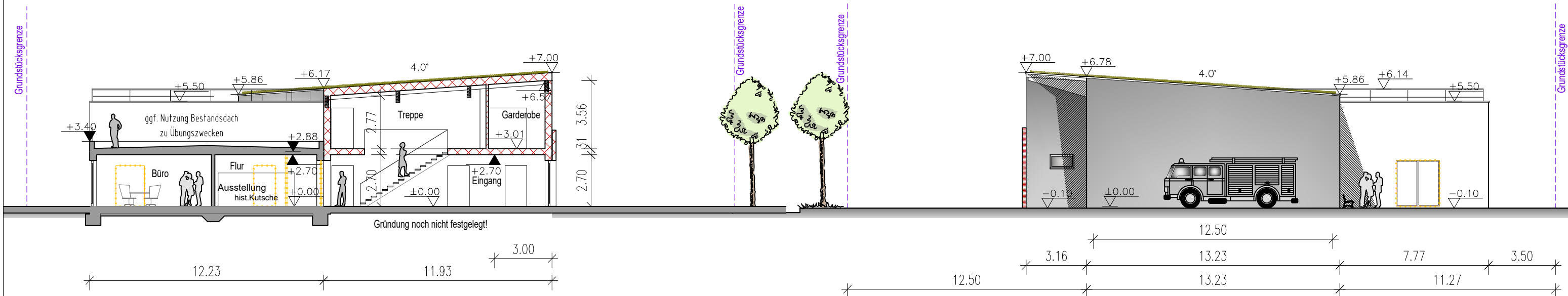
Schnitt B-B
