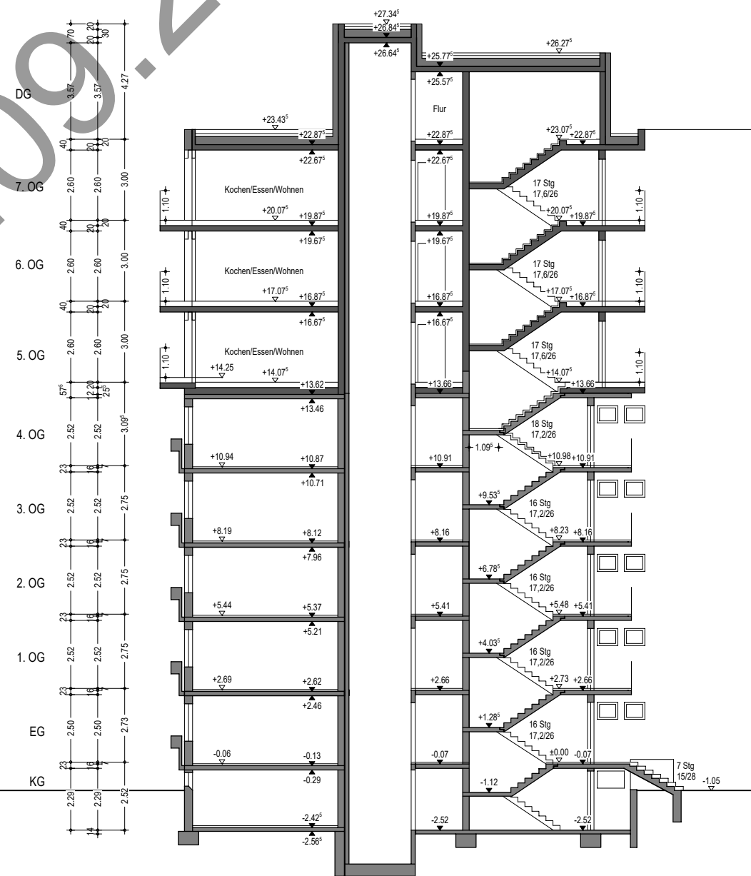
Schnitt A-A
