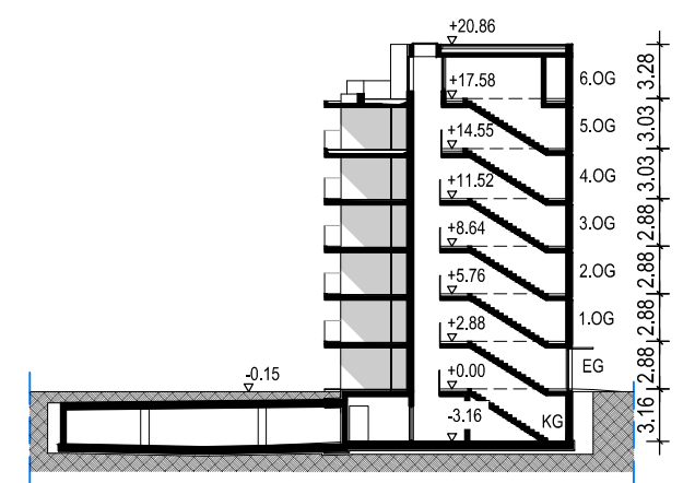
Systemschnitt M 1:500
