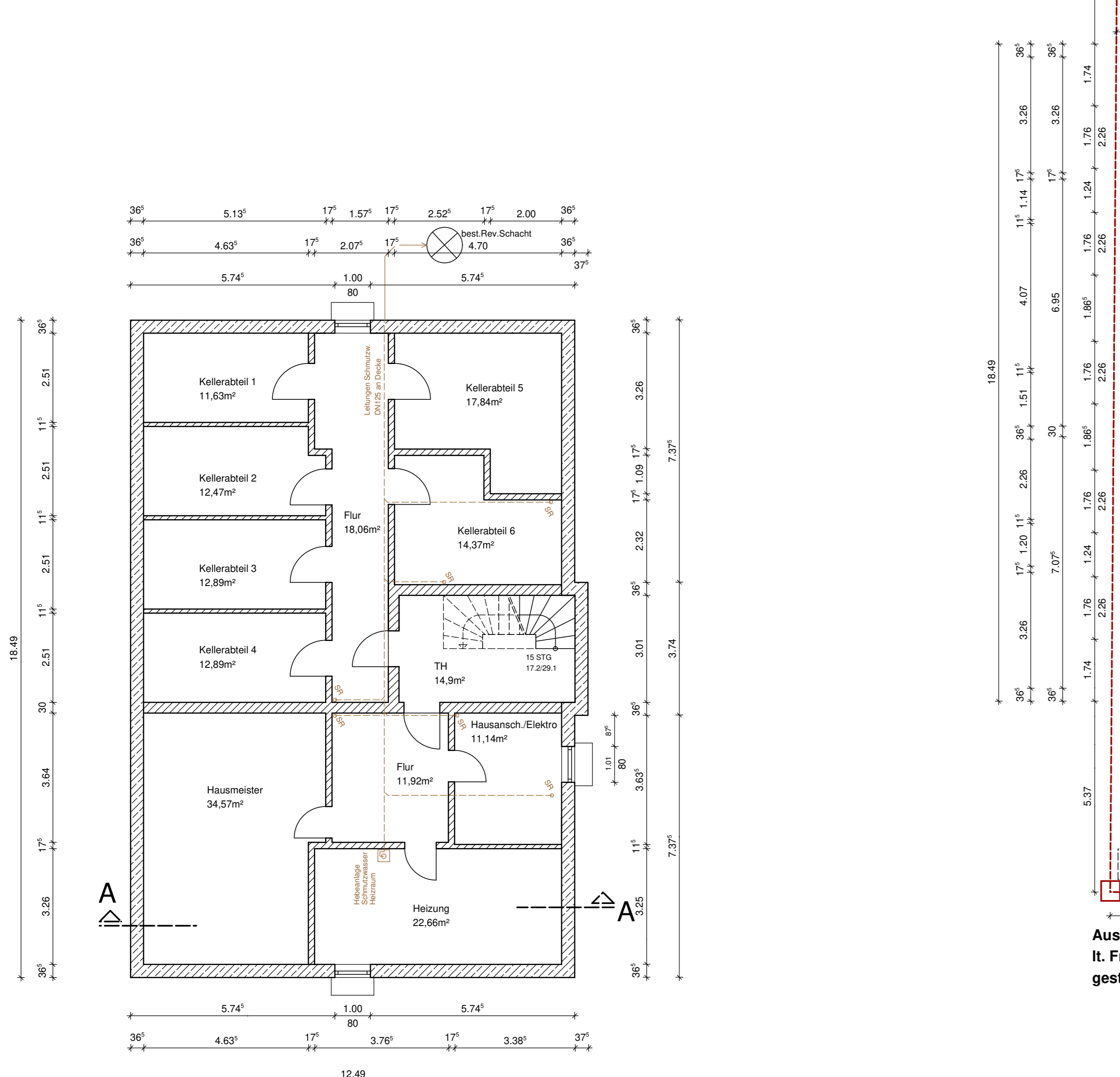
GRUNDRISS UTERGESCHOSS
