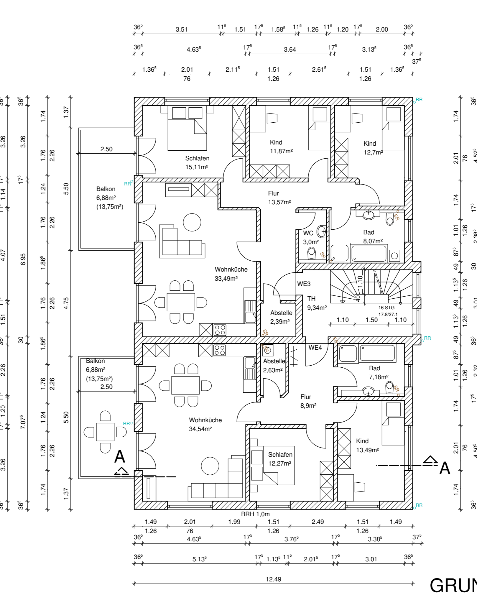
GRUNDRISS OBERGESCHOSS
