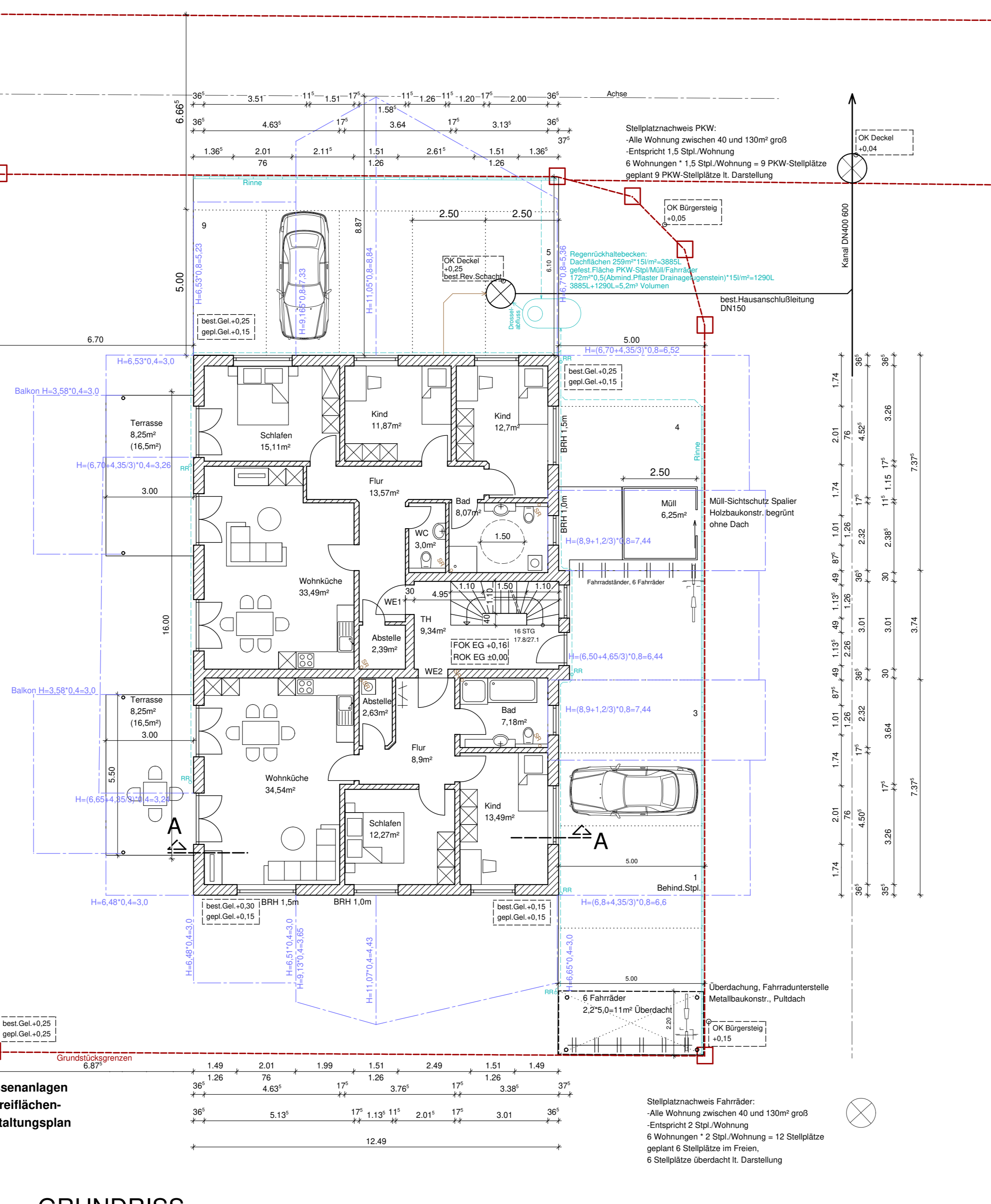
GRUNDRISS ERDGESCHOSS
