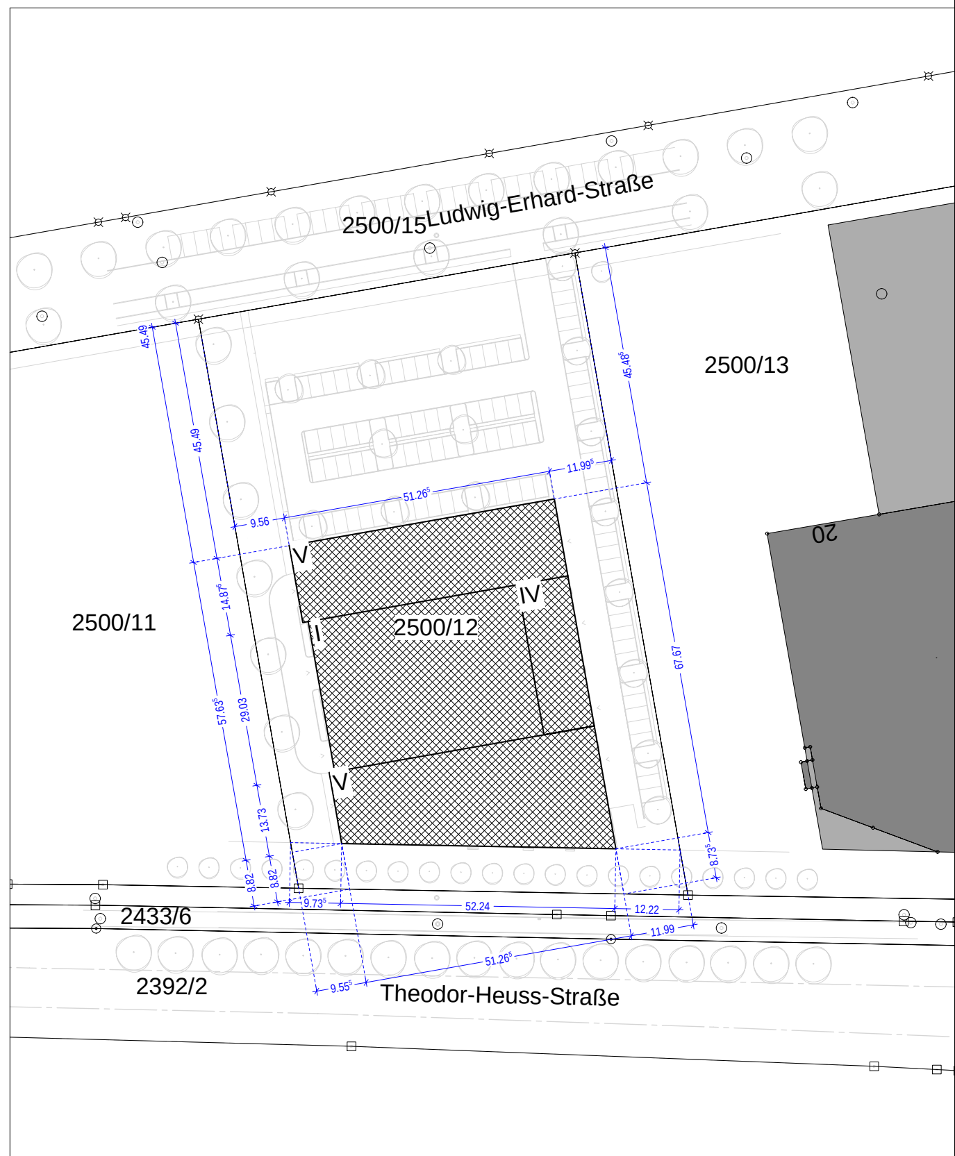
LAGEPLAN M 1/1000
