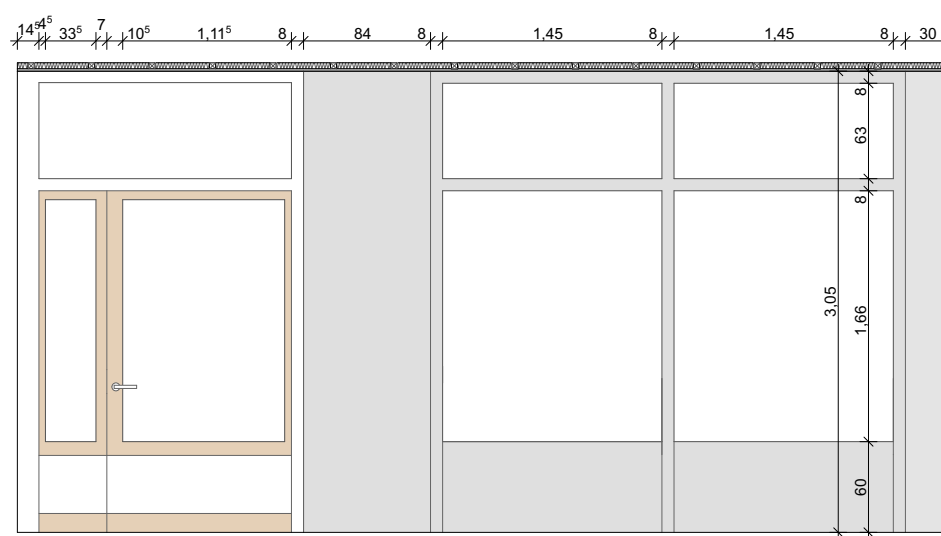
Abwicklung Seite 2 1:50
