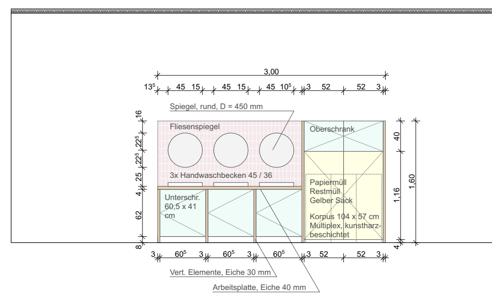
Abwicklung Einbaumöbel, Hinten 1:50
