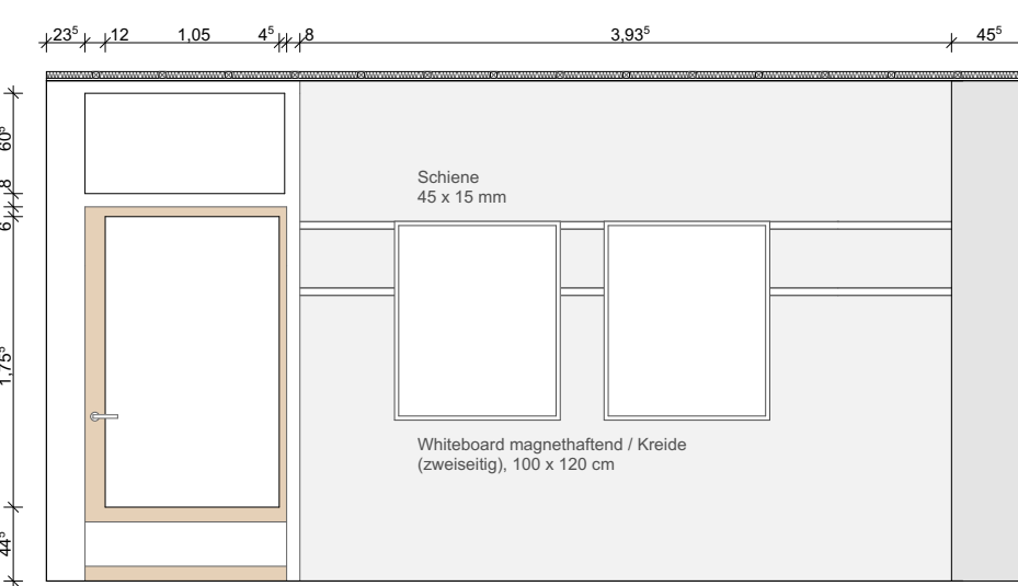
Abwicklung Seite 5 1:50
