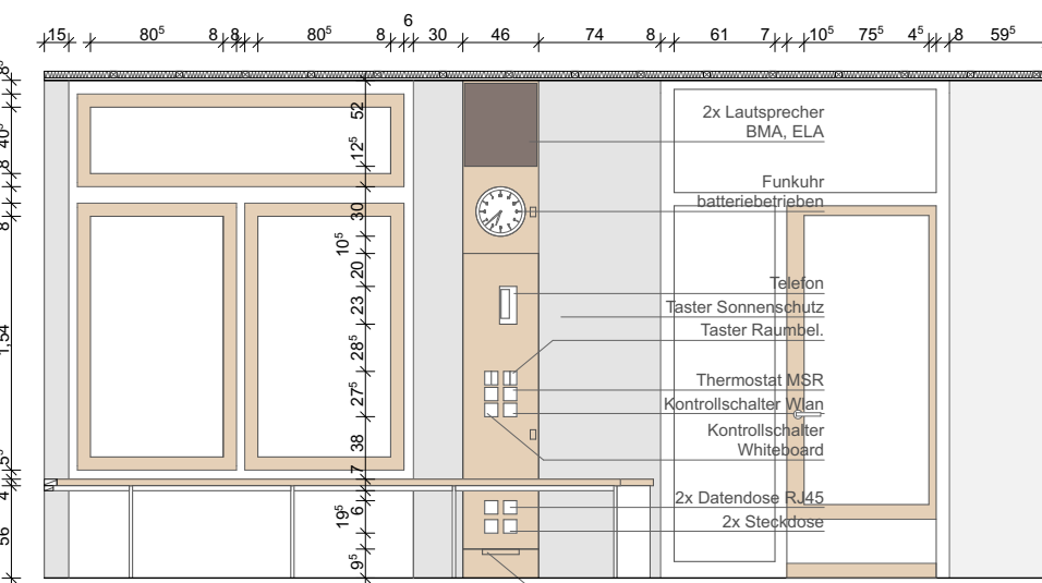
Abwicklung Seite 6 1:50
