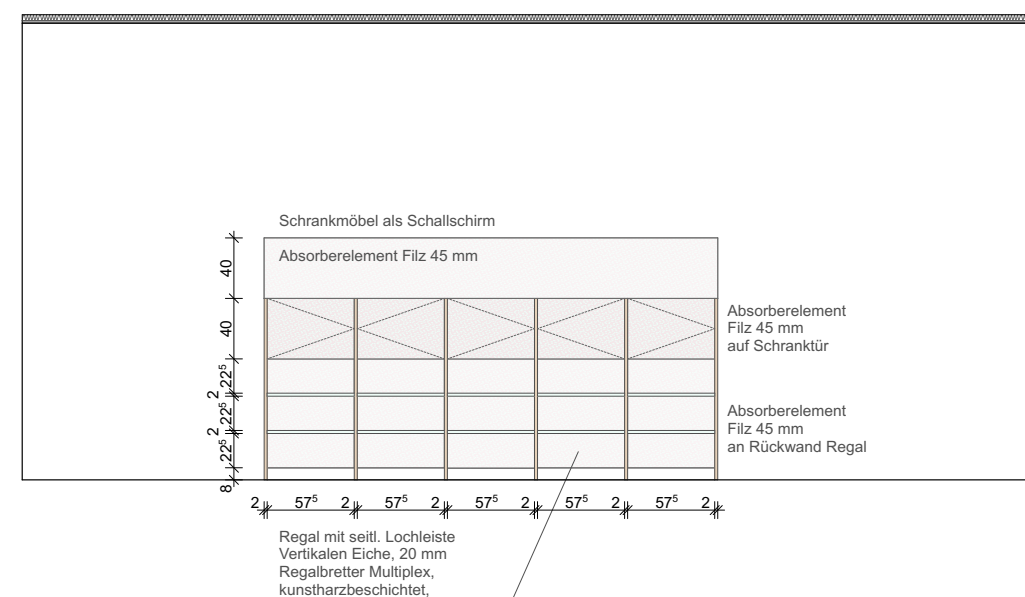
Abwicklung Einbaumöbel, Vorne 1:50
