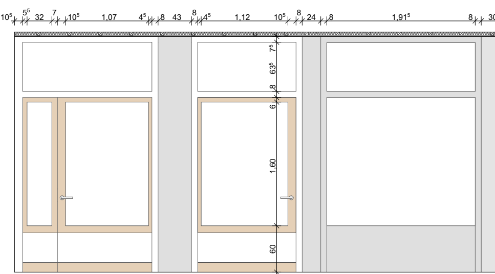
Abwicklung Seite 3 1:50
