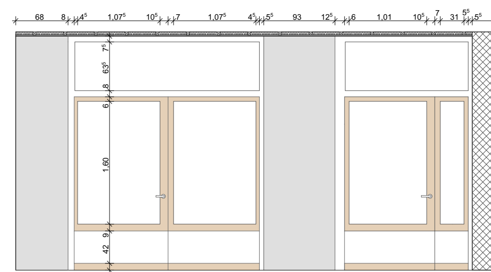
Abwicklung Seite 4 1:50
