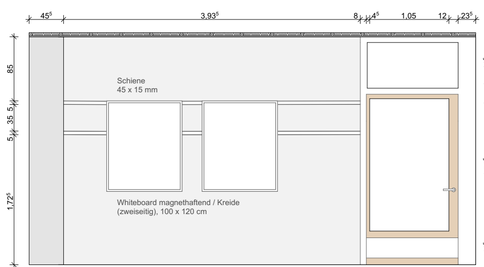
Abwicklung Seite 8 1:50
