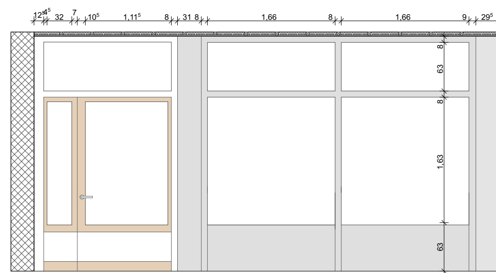
Abwicklung Seite 1 1:50
