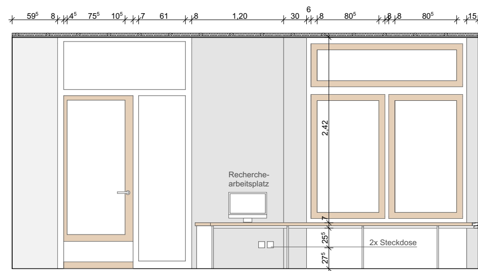
Abwicklung Seite 7 1:50
