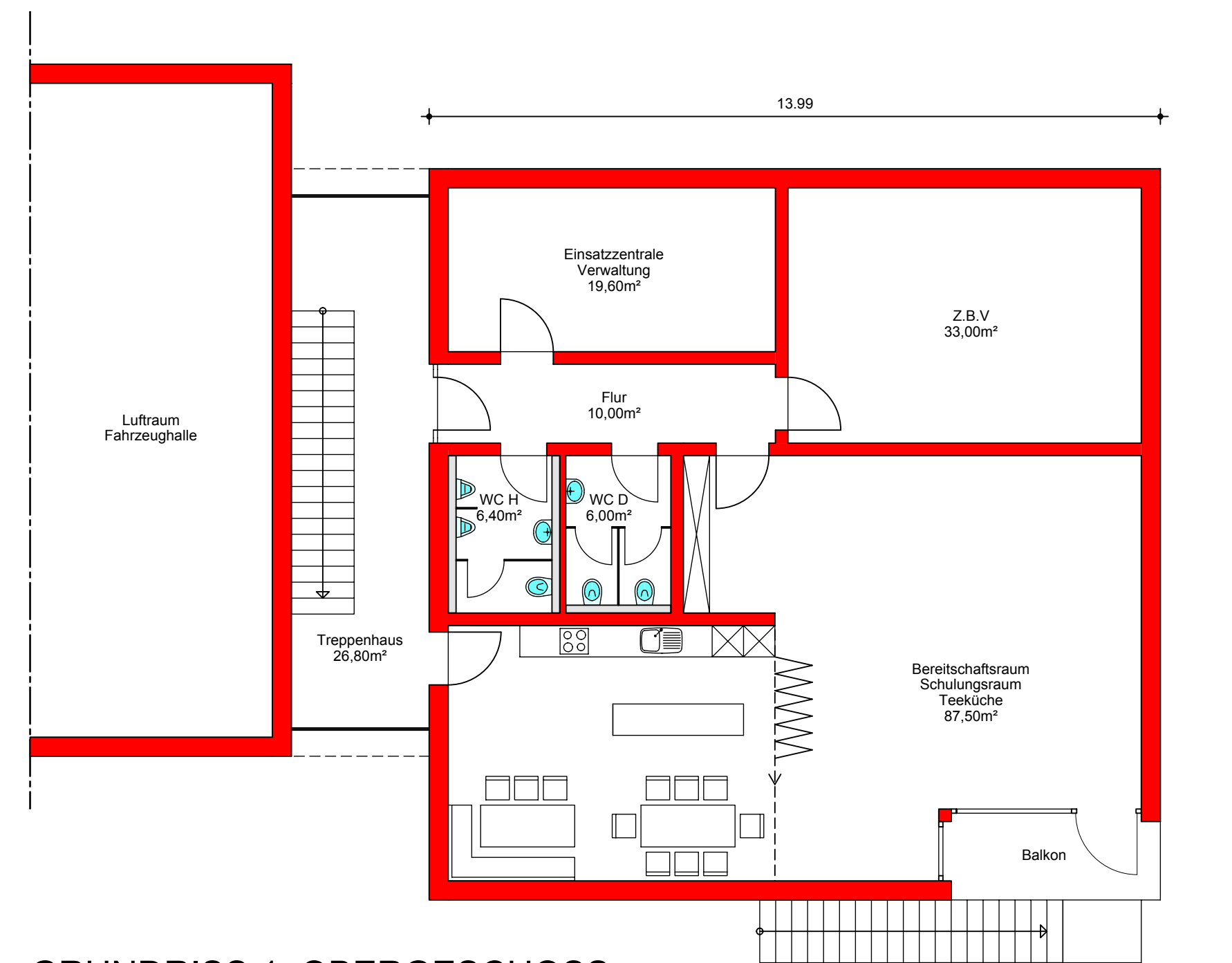
GRUNDRISS 1. OBERGESCHOSS
