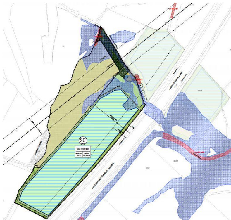
Abb. 9: Ausschnitt aus dem BP „Sondergebiet für PV-Freiflächenanlagen westl. d. A92 südlich Seebach“
