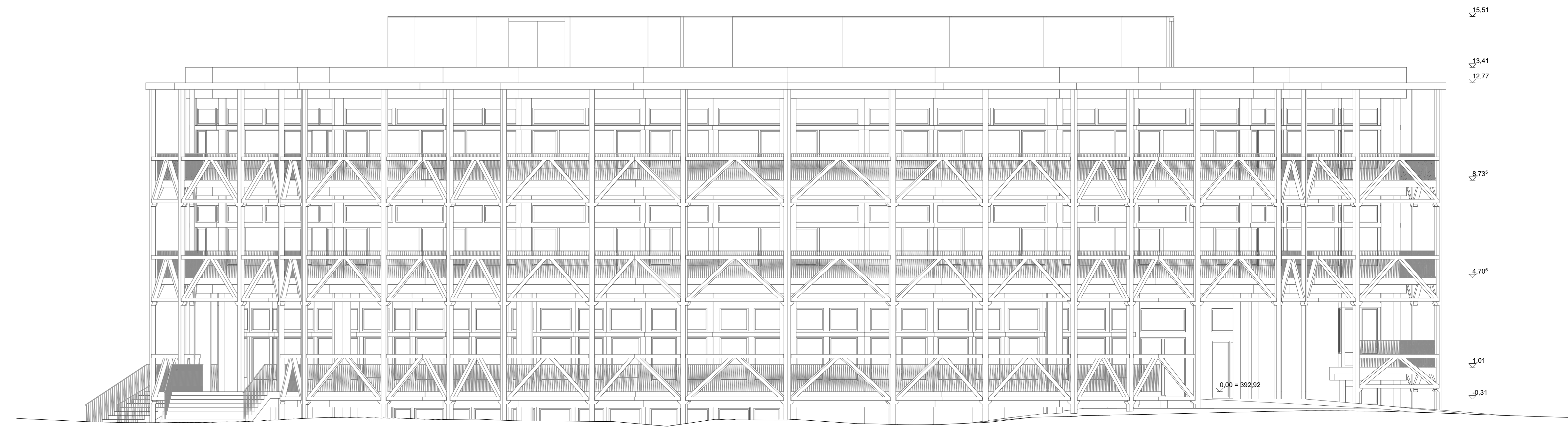
Ansicht West 1:100
