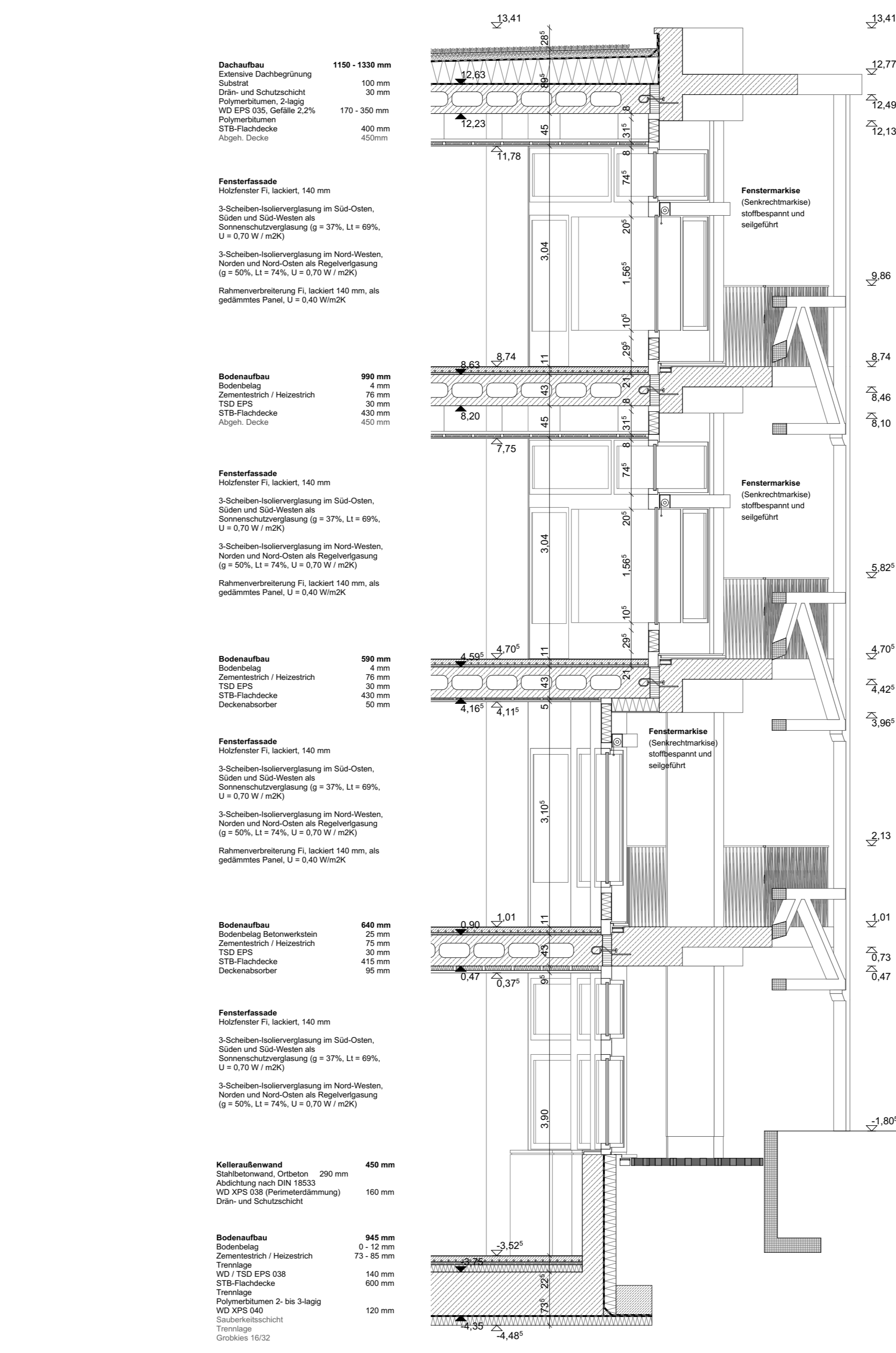
Fassadenschnitt 1:50
