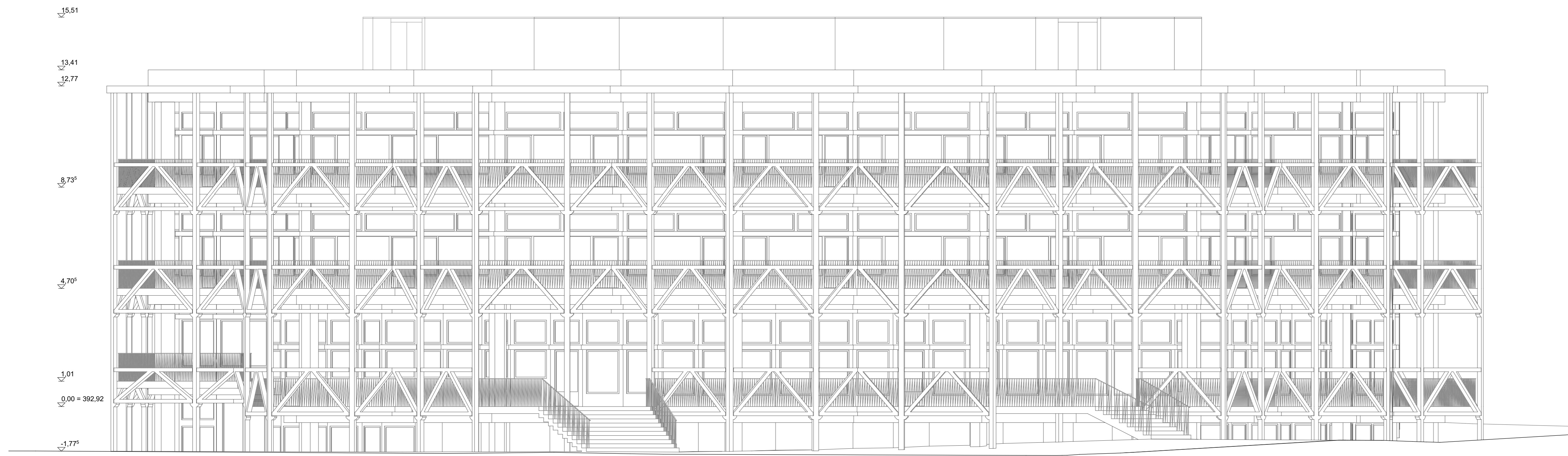
Ansicht Nord 1:100
