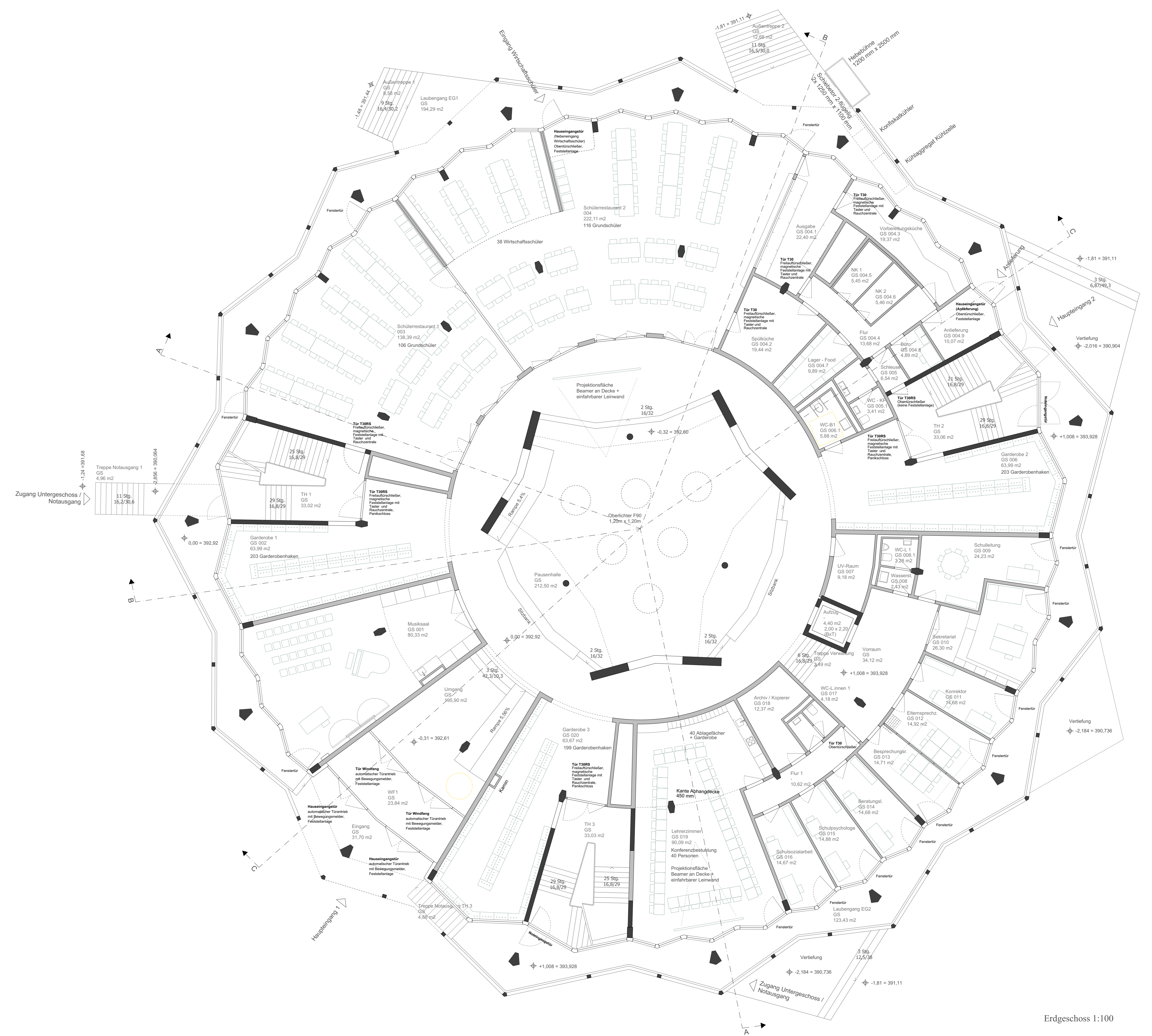
Untergeschoss 1:100
