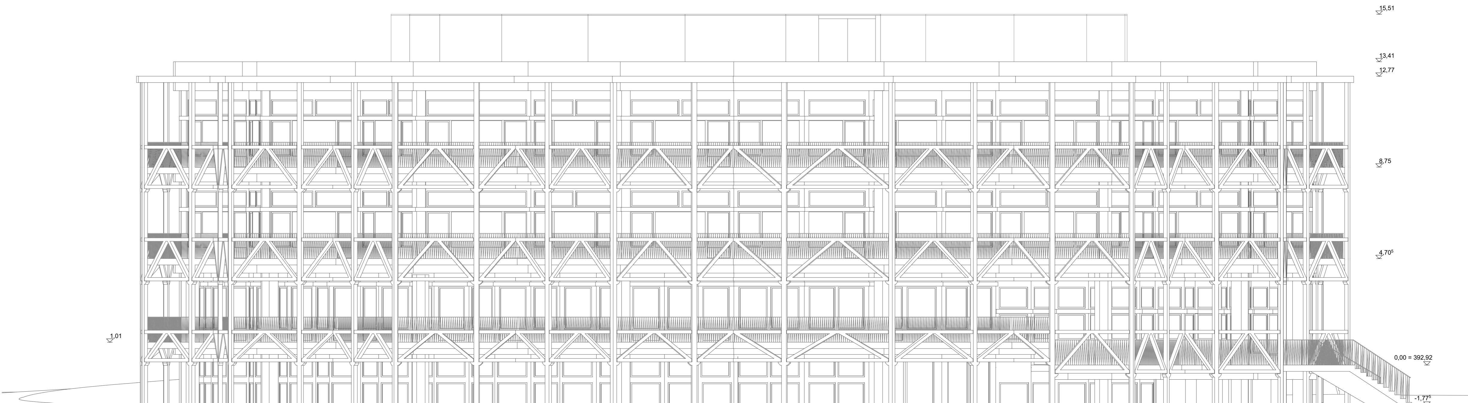
Ansicht Ost 1:100
